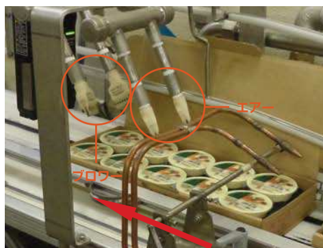
エアで水滴を吹き飛ばす様子
